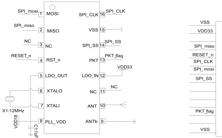
Figure 1. LT8920 典型应用电路
