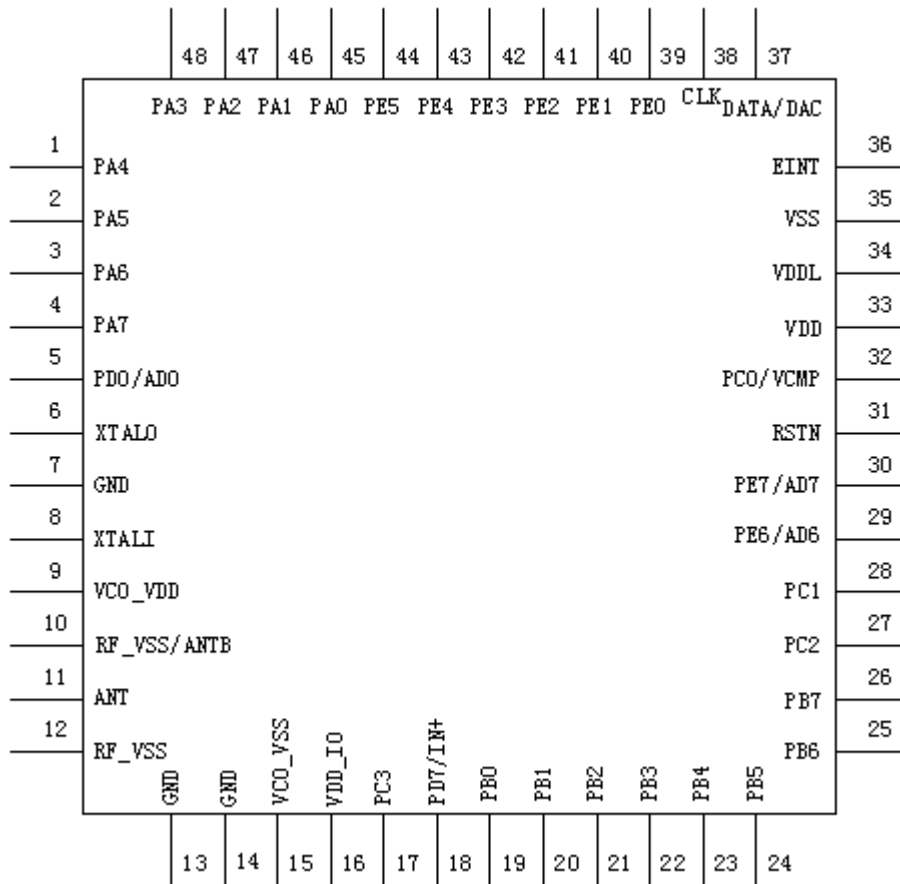
LT6909QP
